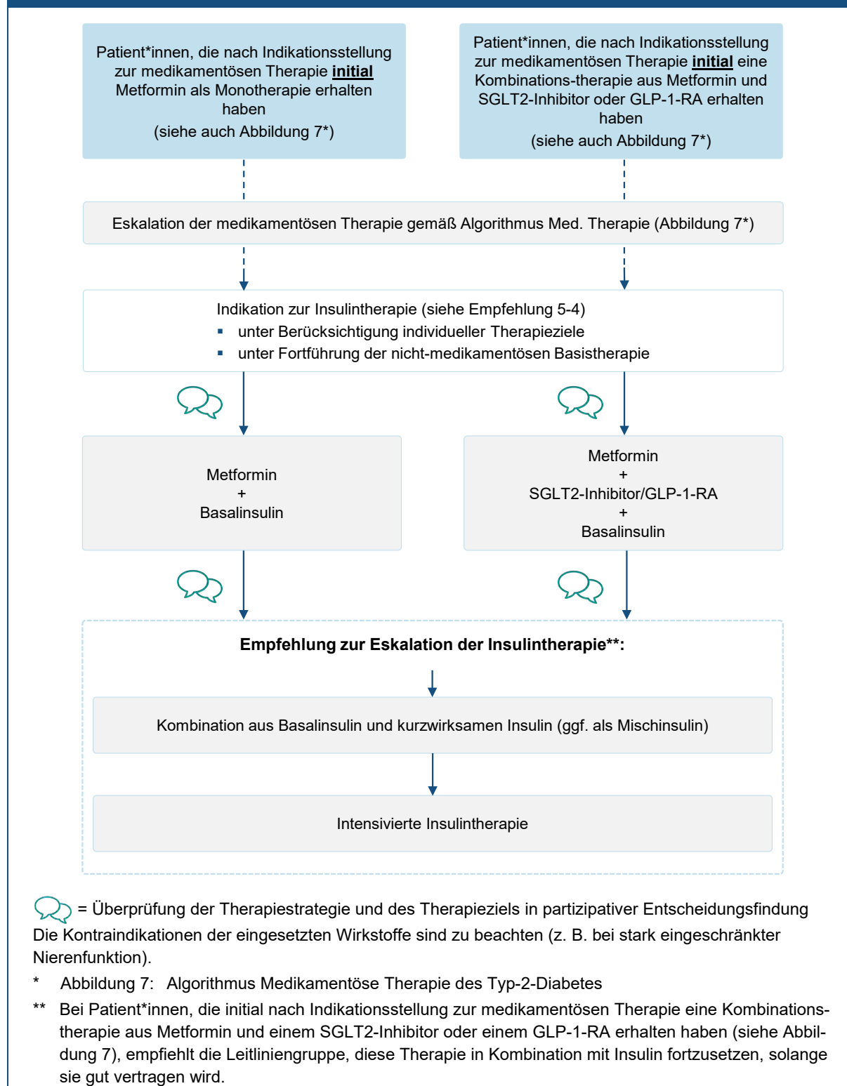
Abbildung 8: Algorithmus Insulintherapie
