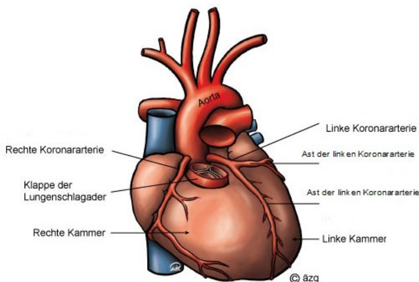
Abbildung 1: Die Herzkranzgefäße
