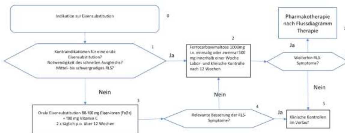
Abbildung 1: Algorithmus Eisensubstitution
